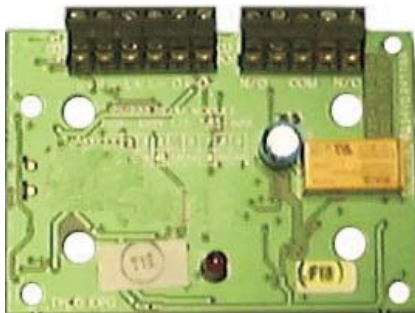
FIG. 1 FC410RIM Modulo relè
